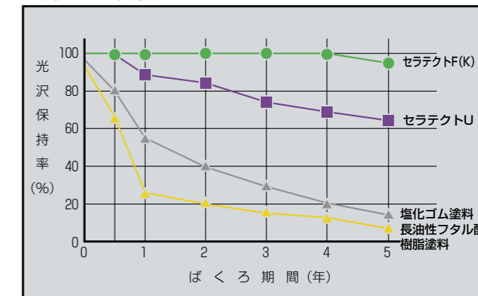
各種上塗塗料の光沢保持性
